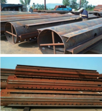
추진관 반제품
