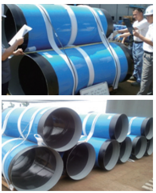
3층PE/폴리우레아
